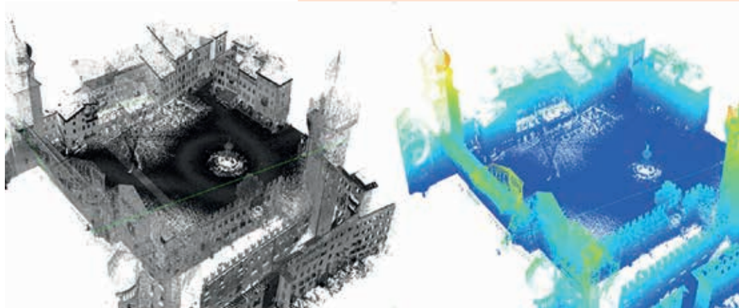
Fig. 1 – Nuvola di punti acquisita da MMS nel centro storico di Trento: mappa di intensità (sinistra) e di altezza (destra).
