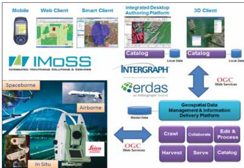
Figura 4 - Architettura di sistema integrata nelle soluzioni IMoSS.
