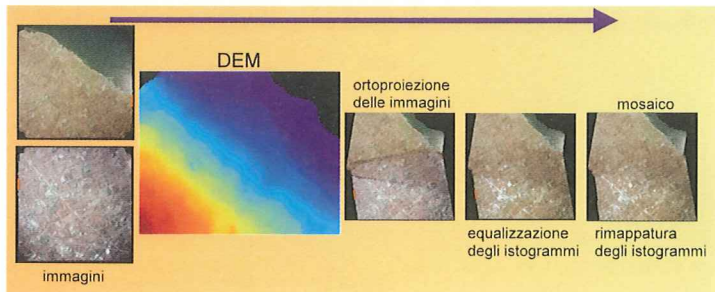
Figura 4 - Esempio di generazione di un ortomosaico con 2 immagini
