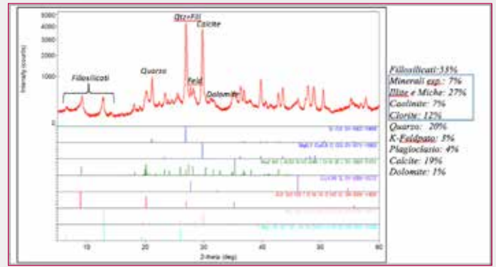
Fig. 13 - Analisi mineralogica del campione LC1S.
