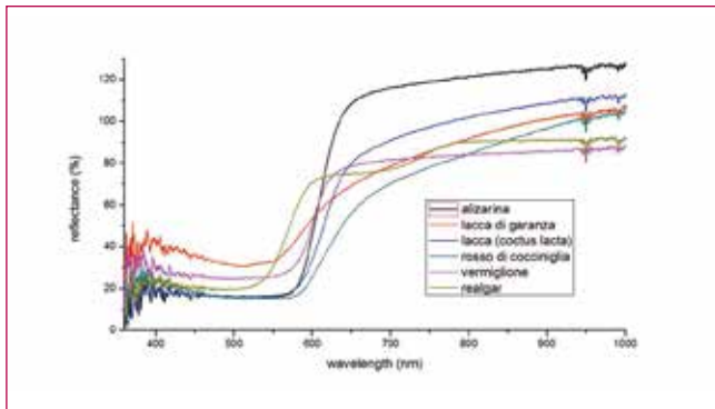
Fig. 10 - Spettri di riflettanza di 6 pigmenti rossi.
