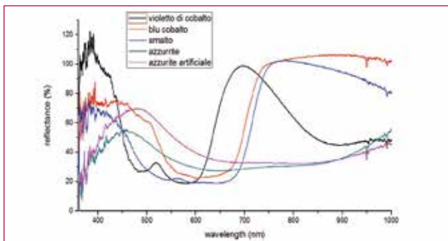
Fig. 5 - Spettri di riflettanza di 5 pigmenti blu.
