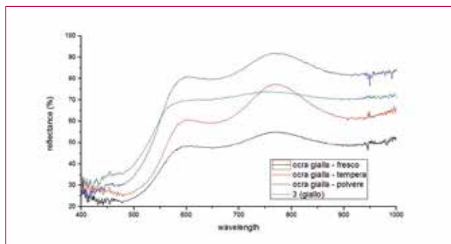
Fig. 20 - Spettri FORS del punto 3 in figura [17] e relativi standard di riferimento dell'ocra gialla applicata con diverse tecniche e in polvere.
