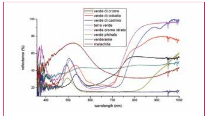
Fig. 7 - Spettri di riflettanza di 8 pigmenti verdi.
