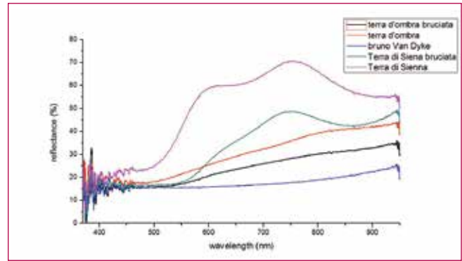
Fig. 12 - Spettri di riflettanza di 5 pigmenti brunì.
