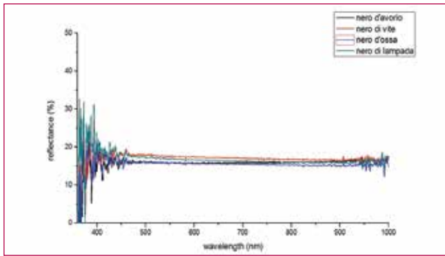
Fig. 4 - Spettri di riflettanza di 4 pigmenti neri.
