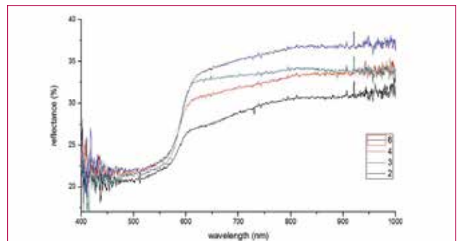
Fig. 18 - Spettri FORS del punto 1 in figura [17] e relativi standard di riferimento dello smalto applicato con diverse tecniche e in polvere.
