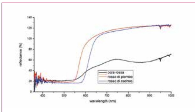
Fig. 11 - Spettri di riflettanza di 6 pigmenti rossi.
