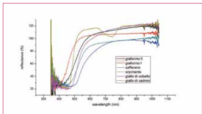
Fig. 8 - Spettri di riflettanza di 6 pigmenti gialli.
