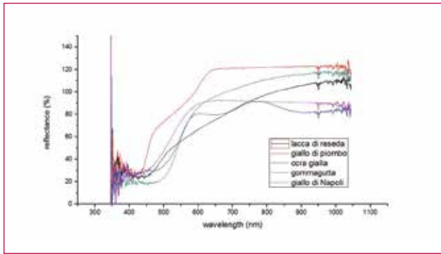
Fig. 9 - Spettri di riflettanza di 5 pigmenti gialli.
