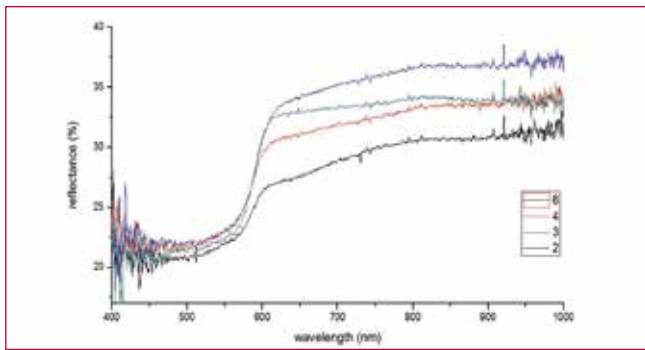
Fig. 15 - Spettri FORS dei punti 2, 4, 6 (area ritoccata) e 3 (area originale) sull'ala dell'angelo in alto a sinistra.
