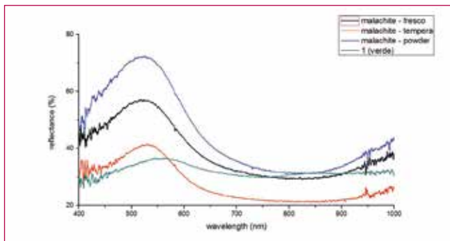
Fig. 22 - Spettri FORS del punto 1 della area in figura [21] e relativi standard di riferimento della malachite applicato con diverse tecniche e in polvere.
