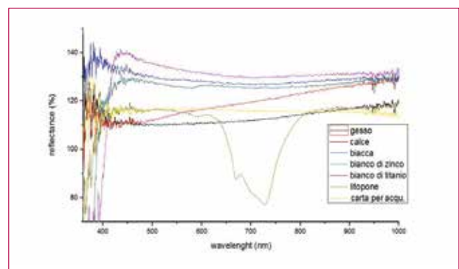
Fig. 3 - Spettri di riflettanza di 6 pigmenti bianchi e della carta per acquerello.
