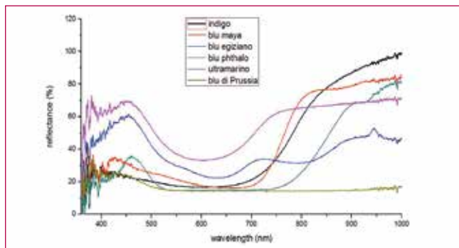
Fig. 6 - Spettri di riflettanza di 6 pigmenti blu.
