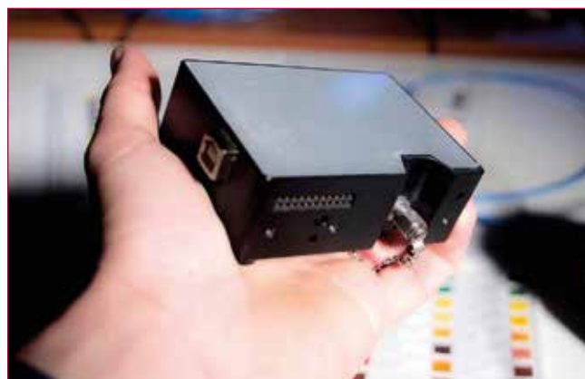
Fig. 2 - Lo spettrometro USB4000, parte del sistema FORS testato in questo articolo, sta tutto in una mano e pesa meno di 200 gr.
