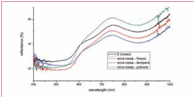
Fig. 19 - Spettri FORS del punto 2 in figura [17] e relativi standard di riferimento dell'ocra rossa applicata con diverse tecniche e in polvere.
